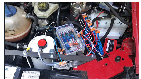
Beispiel eines HHO-Systems, Einbau in einem VW T4, Baujahr 1998.
